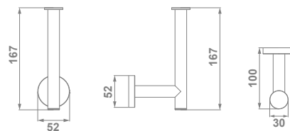
€/u 53154 PORTARROLLOS DE RESERVA 34,0
