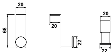
53142 PERCHA COLGANTE €/u 40,3 ● 02 Negro ● 00 Cromo
