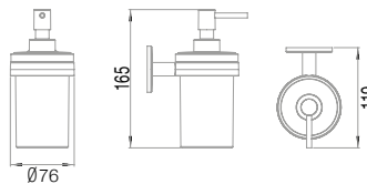
53160 DOSIFICADOR DE VIDRIO €/u 48,2
