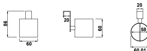
53145 SOPORTE PLANCHA PELO COLGANTE €/u 50,9 ● 00 Cromo ● 02 Negro
