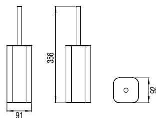
53212 ESCOBILLERO DE SUELO 00 Cromo €/u 95,2
