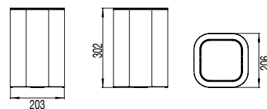
53225 PAPELERA 5L INOX BRILLO 53213 PAPELERA 5L CROMO 00 Cromo €/u 142,1 €/u 181,7
