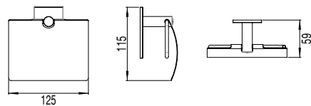
52991 PORTARROLLO CON TAPA 54,4 €/u ● 00 Cromo ○ 01 Blanco ● 02 Negro
