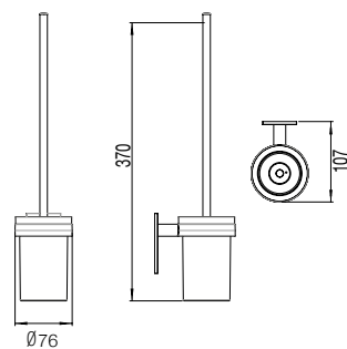
52982 ESCOBILLERO DE PARED 70,5 €/u ● 00 Cromo ○ 01 Blanco ● 02 Negro
