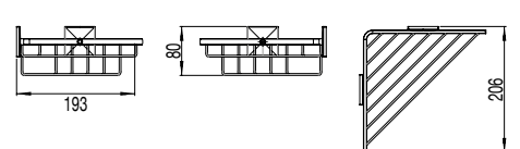
53199 CONTENEDOR DE DUCHA DE RINCÓN 20x21x8 74,2 ● 00 Cromo
